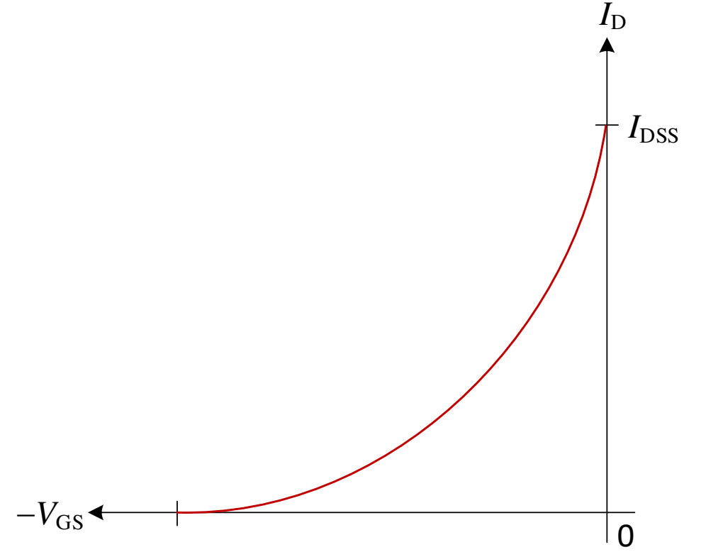
Şekil 9 n -kanal JFET için transfer karakteristik eğrisi.
