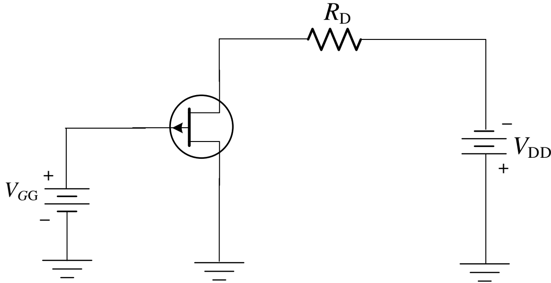
Şekil 7 p-kanal JFET'in beslenmesi. V_{GG} nin pozitif ve V_{DD} nin negatif olması dışında p-kanal JFET'in çalışma işlemi n-kanalıinkiyile aynıdır.
